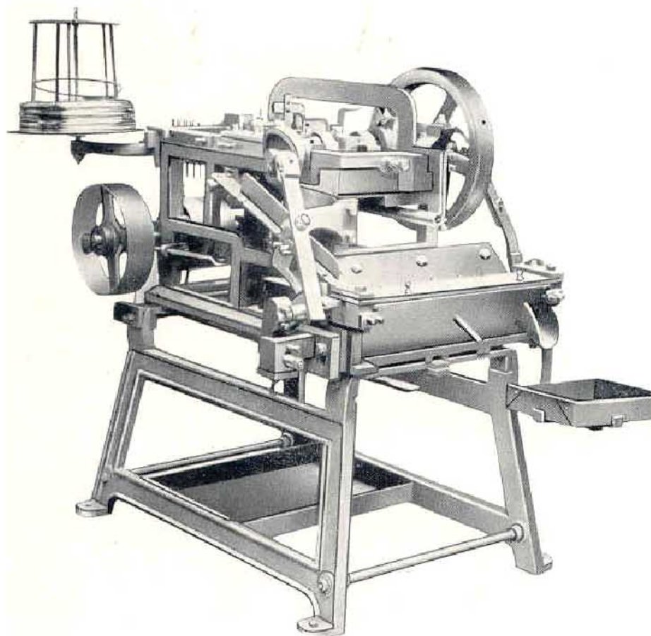
Máquina de alfileres utilizada desde 1924 al 1965 Pin making machine used from 1924 till 1965
